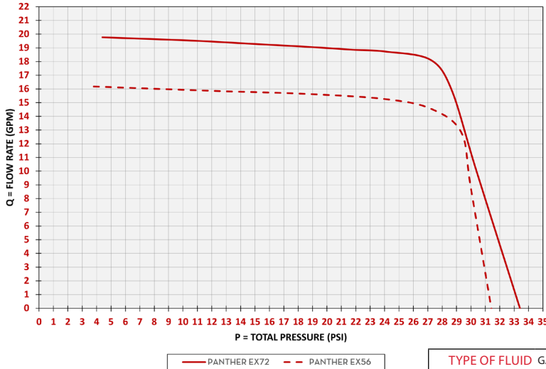
PANTHER EX 56 / PANTHER EX 72
